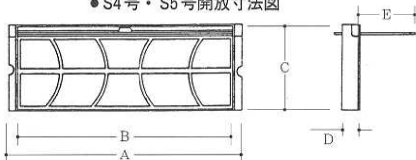
●S4号・S5号開放寸法図
