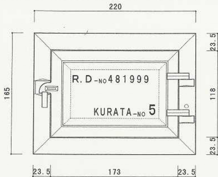
閉鎖時正面図
