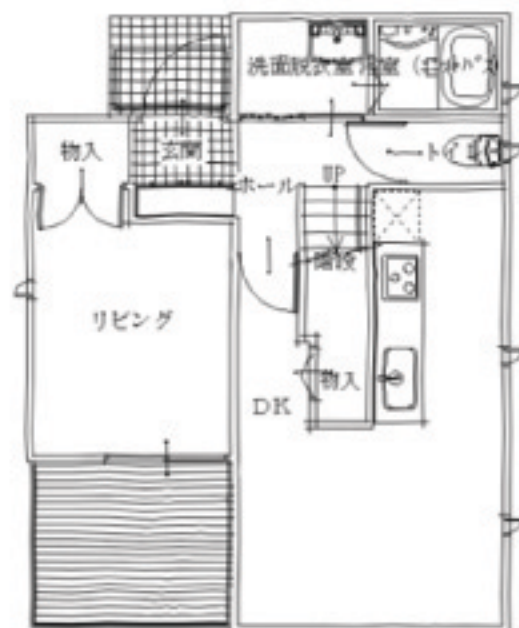
1階平面図
